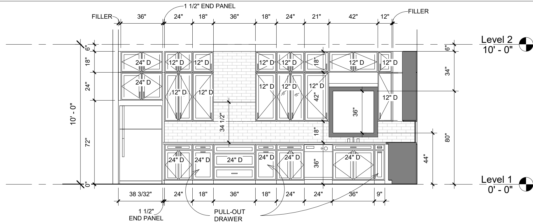
① ELE 1 1/4" = 1'-0"
