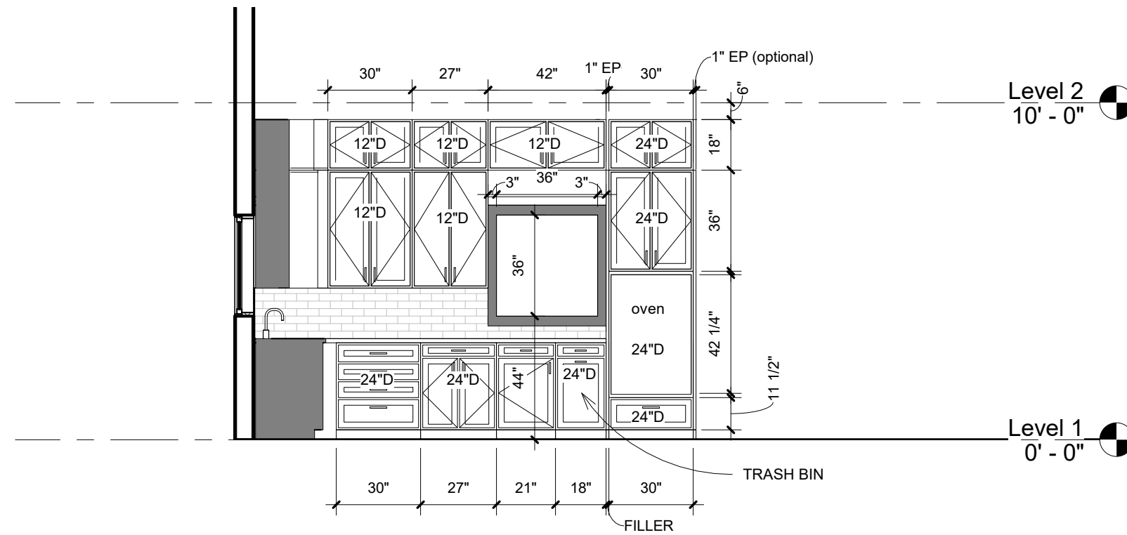
② ELE 2 1/4" = 1'-0"
